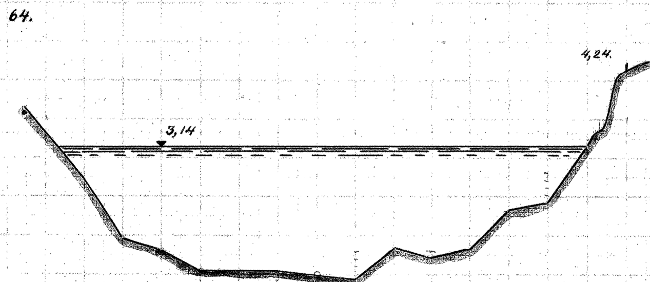
MÅLESTOK FOR LÆNGDER 1:200.
