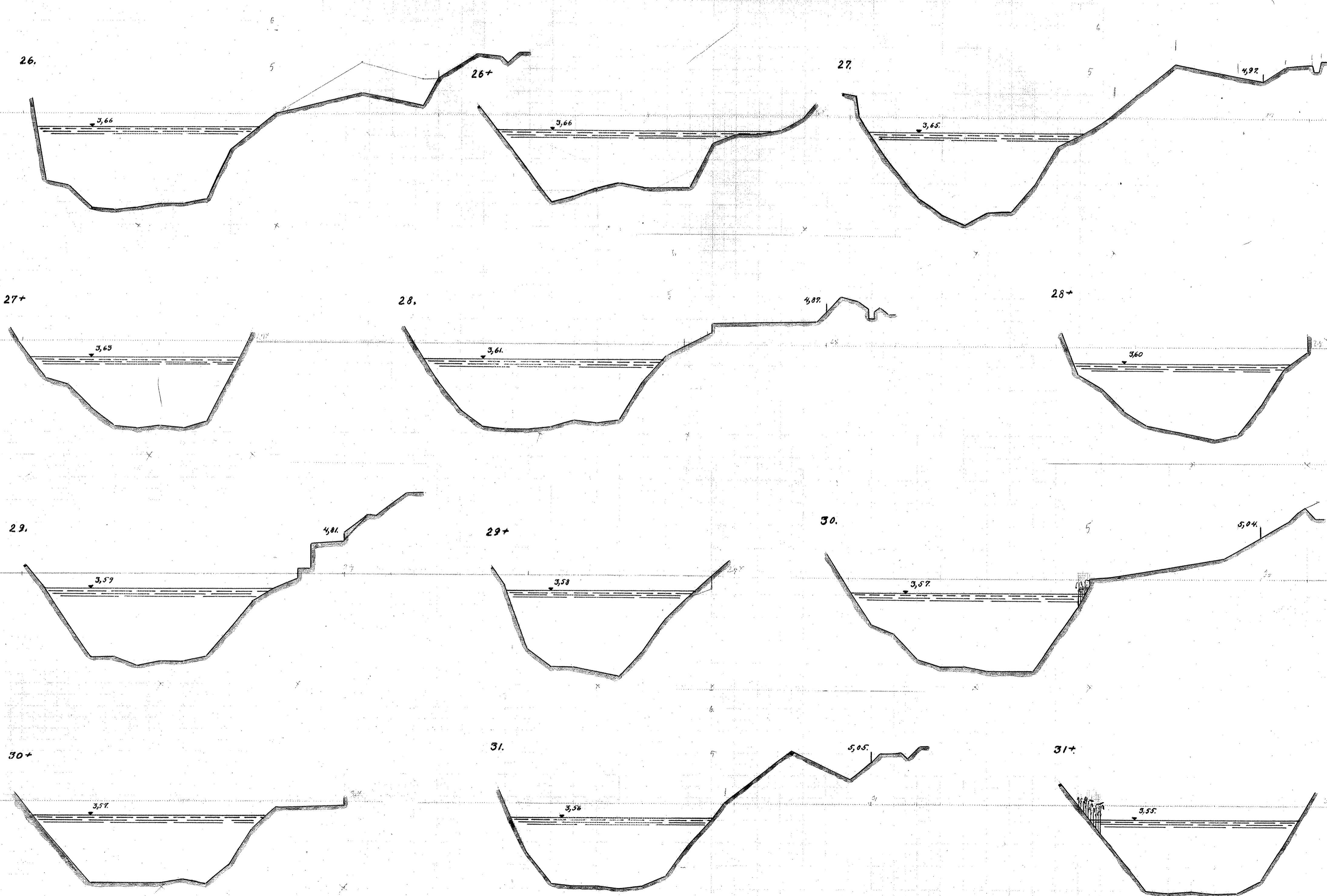
MAALESTOK FOR LÆNGDER. 1:200.
