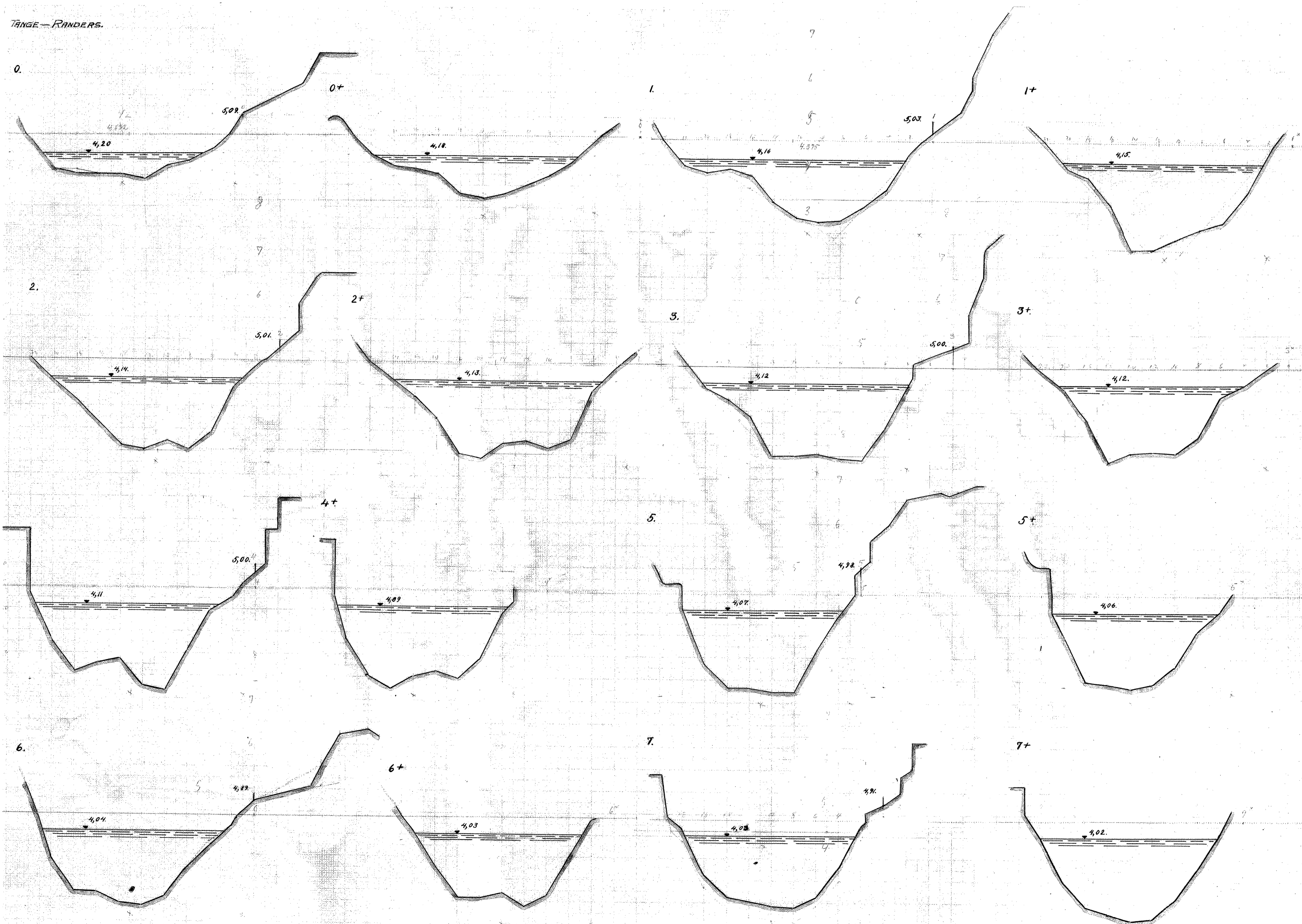
MÅLESTOK FOR LÆNGDER 1:200.
