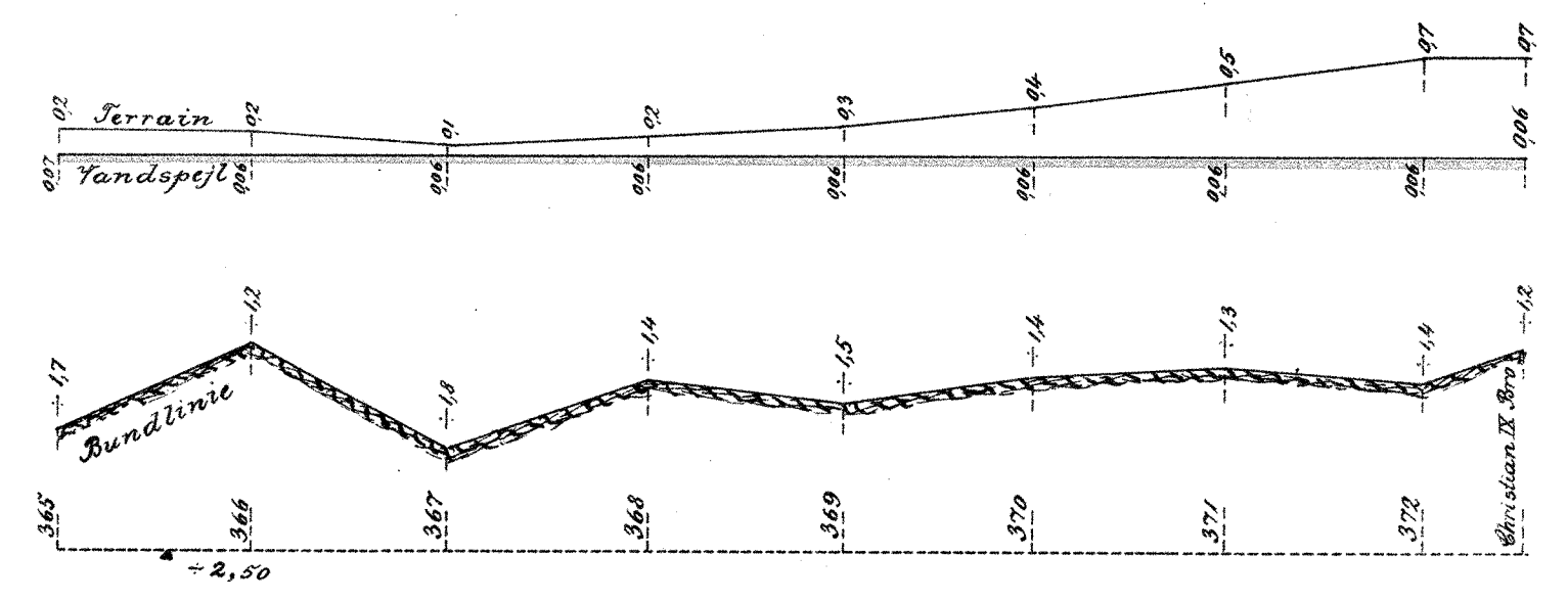
Langdeprofil 365 - Christian IX Bro. (nordre Løb).
