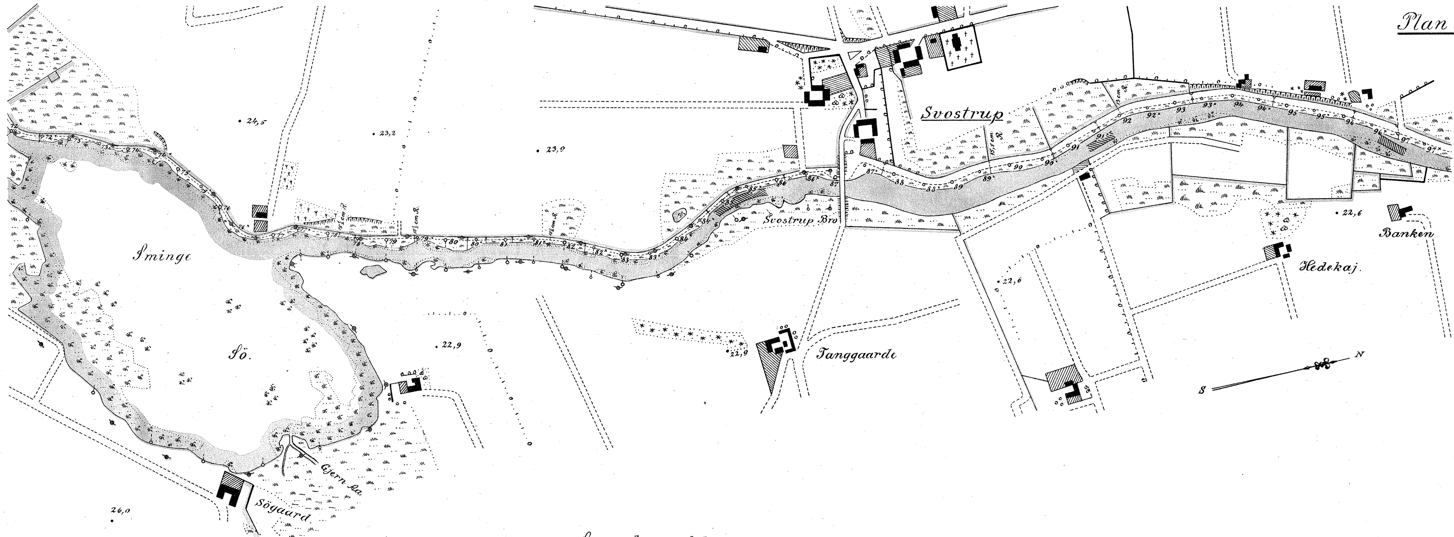
Langdeprofil 72°-97°
