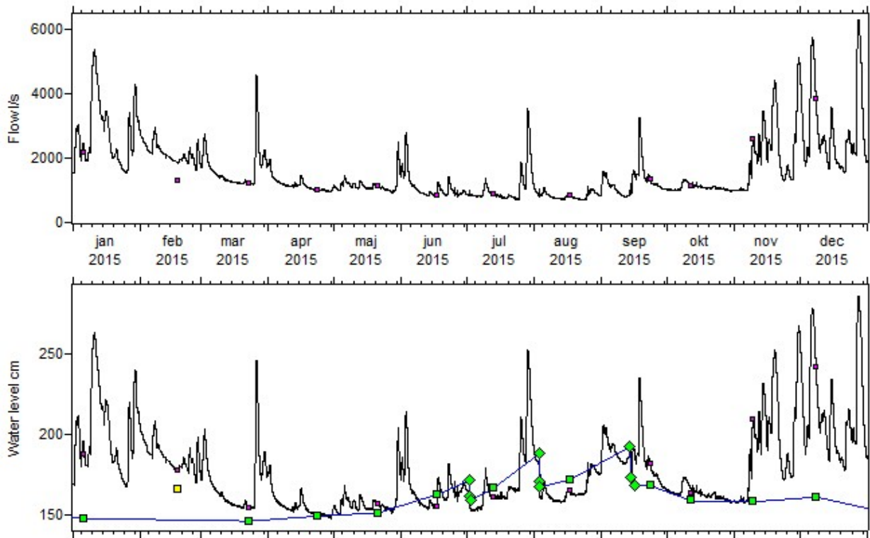
Figur 3.1. Trend Å, vandføring og vandstand 2015. Blå kurve: Kontrolvandstand ved en konstant kontrolvandføring på 1000 l/sek. Udviklingen i grødens betydning for vandføringsevnen kan direkte aflæses af kontrolvandstanden. Der kan identificeres 3 grødeskæringer i løbet af året, hvor kontrolvandstanden falder momentant med mellem 10 og 25 cm. Grønne firkanter angiver målte vandføringsværdier, hvoraf de, der står på spidsen, er estimerede værdier til støtte for beregningen
