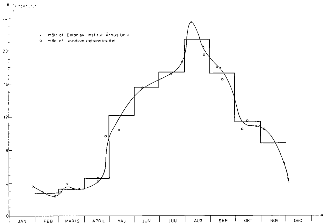
Figur 3.5 Overfladevandtemperatur, Mossø - 1975.
