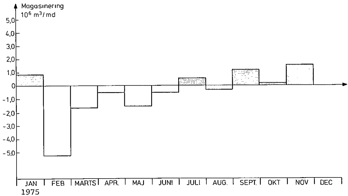
Figur 2.2 Magasinering, Mossø - 1975.
