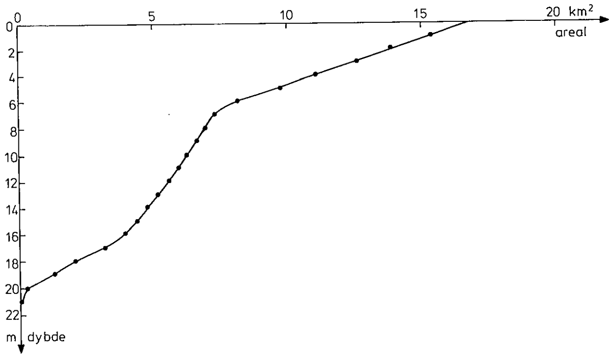
Figur 3.1 Hypsografisk kurve, Mossø.
