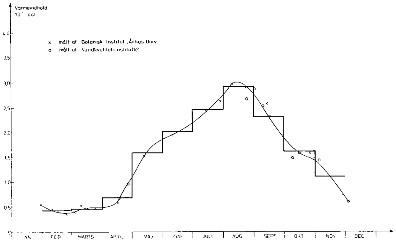
Figur 3.2 Varmeindhold, Mossø - 1975.
