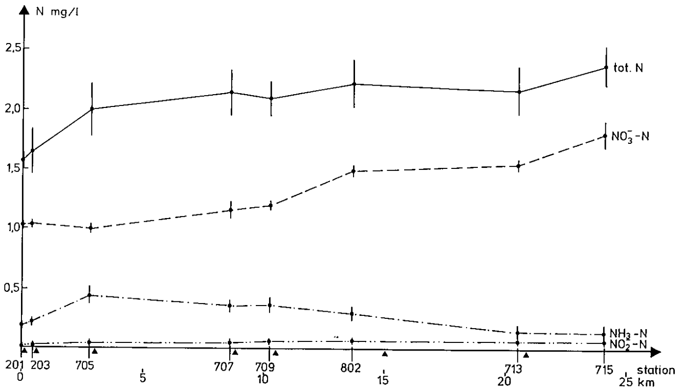
Figur 3.4 Kvalstofkoncentrationer på Gudenastrækningen Tørring - Bredvad mølle den 25. - 26. juni 1974. De lodrette linier i hver station viser standardafvigelse.
