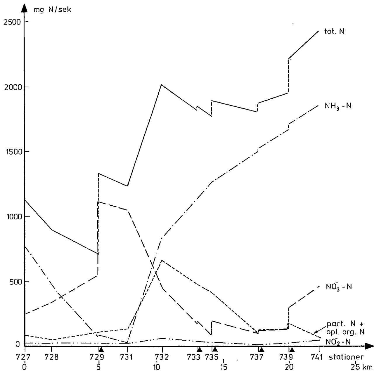
Figur 7.4 Transporten af kvælstof ned ad Hadsten lilleå målt den 29. - 30. august 1974. De lodrette spring på kurverne viser sidetiløbets bidrag.
