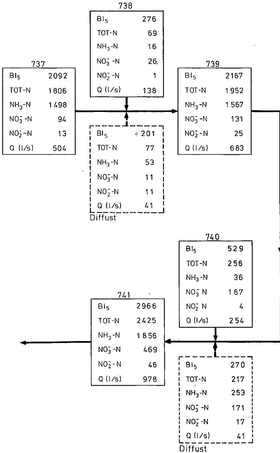
Figur 7.8 Massebalance for BI 5 og kvælstof i Hadsten lilleå på grundlag af målinger den 29. - 30. august 1974.
