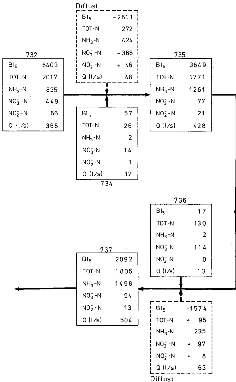
Figur 7.7 Massebalance for BI 5 og kvælstof i Hadsten lilleå (732), (735) og (737) og de to tilløb Vissingø bæk (734) og Faurskov bæk (736). Enheder er mg/sek. Tallene er målt den 29. - 30. august 1974.
